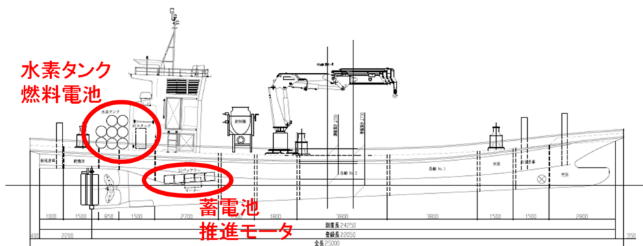
図1. 水素燃料電池マグロ養殖作業船の一般配置図
