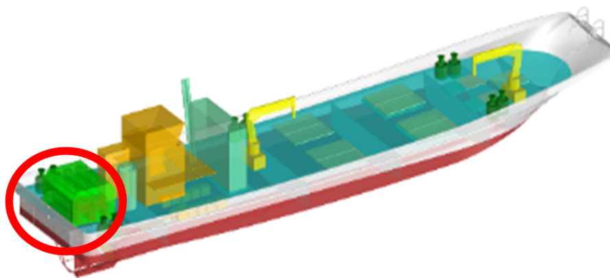
図2. コンテナ型水素燃料電池システム (○ 部分) による 既存の養殖作業船の電動化
