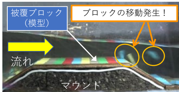
図2. 水理模型実験の様子
