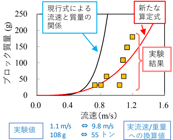
図3. ブロック質量と移動開始時流速との関係の例
