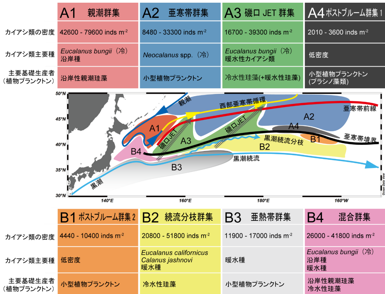
図 1. カイアシ類群集の地理分布及び各群集の特徴。地理分布は結果を基に作成。種名の隣に(冷)と書かれた種類は冷水種、それ以外は暖水種であることを示す。ポストブルーム群集 1 (A4) と 2 (B1) は、植物プランクトンの増加が終了し、A3 と B2 から遷移した群集であると考えている。
