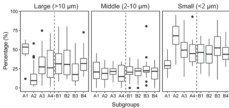
図2. 各群集におけるサイズ分画したクロロフィル a 濃度。どのようなサイズの植物プランクトンが多いのかを示してしている。亜寒帯群集 (A2) や亜熱帯群集 (B3) では小型の植物プランクトン (Small) の割合が他の群集に比べて高く、その他の群集では大型 (Large) の割合が高い。
