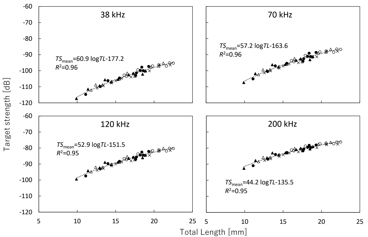
図 2．ツノナシオキアミの全長（TL）と姿勢平均TSの関係
