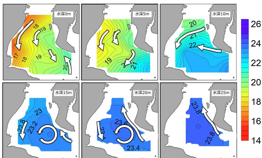
図3 密度の水平分布から推定した流動構造.
