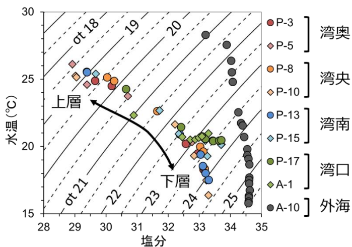
図2 TS-ダイアグラム. 5m ごとにプロットした.
