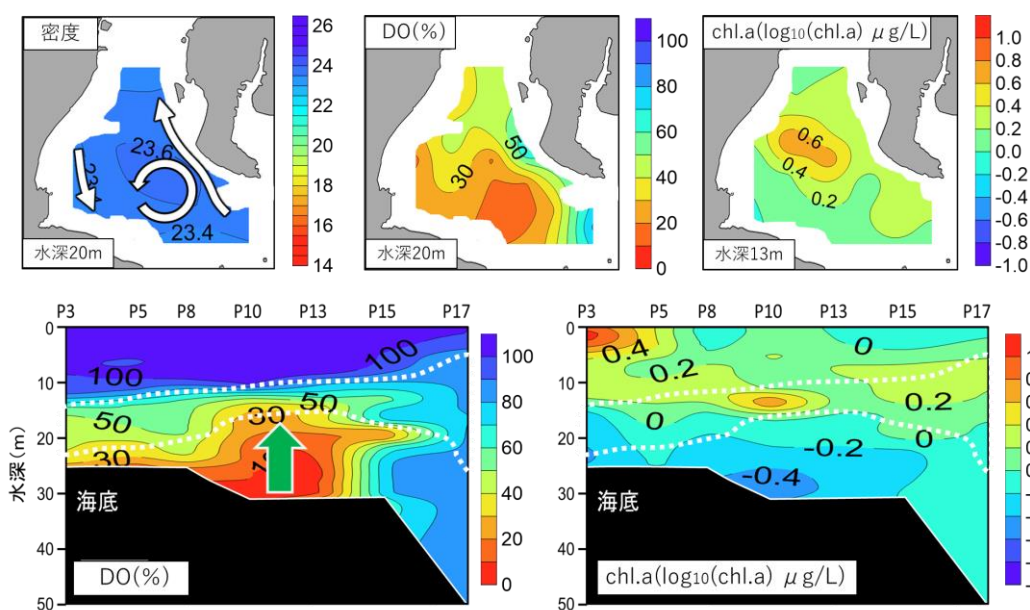
図4 水深 10m と 15m の水平分布図と南北断面図. 南北断面図で白色の破線で囲まれた部分は、湾口部混合水 (ot22.5~23.5) の分布を示す.
